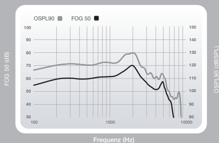
Wiedergabekurven für OSPL90 (grau) und Full-On Gain (schwarz) für die Geräte Muse CIC mit der Matrix 130/70
