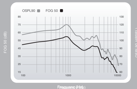
Wiedergabekurven für OSPL90 (grau) und Full-On Gain (schwarz) für das Gerät Muse mini HdO 312 mit Mikroschlauch
